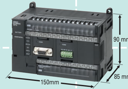
CP1L-M40D
