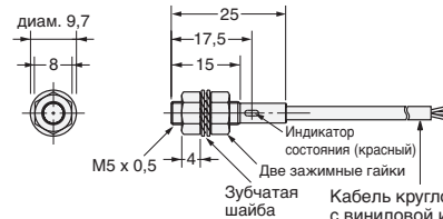
Рис. 3 : E2E-X1□□
