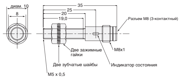
Рис. 36 : E2E-X1□□-M5
