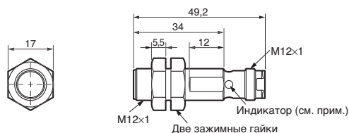
E2A3-M12KS06-M1-□□
