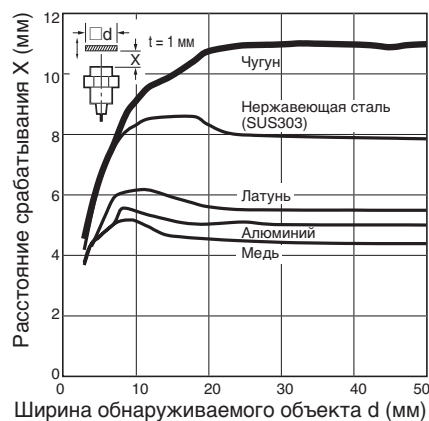
E2A3-M18KS11
