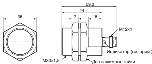
E2A3-M30KS20-M1-□□
