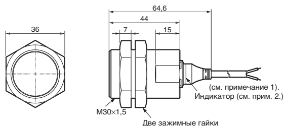
E2A3-M30KS20-WP-□□
