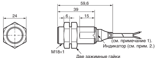
E2A3-M18KS11-WP-□□
