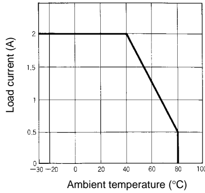
G3R-102□, G3RD-X02□, G3R-202□
