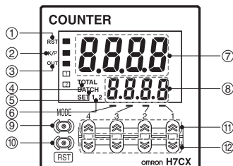
Вид спереди модели с 4-символьным дисплеем
